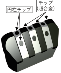
スタミナビット(SG30種)
