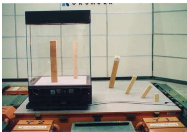
免震展示ケースの振動実験
