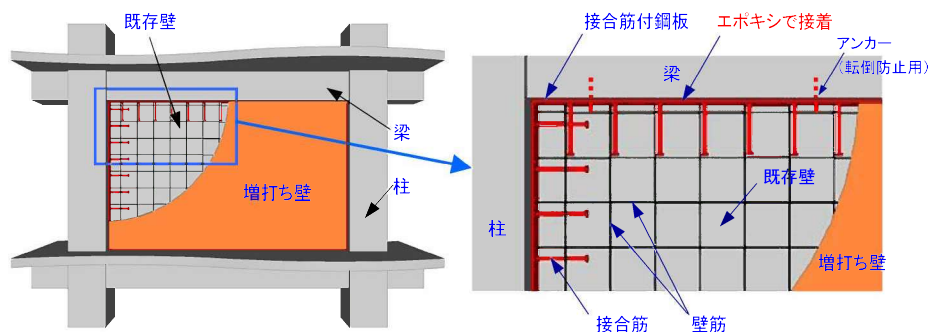
工法の概要
