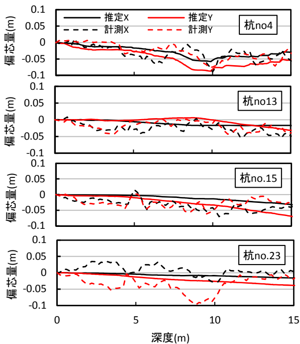
杭偏心量の推定曲線と孔壁測定との比較
