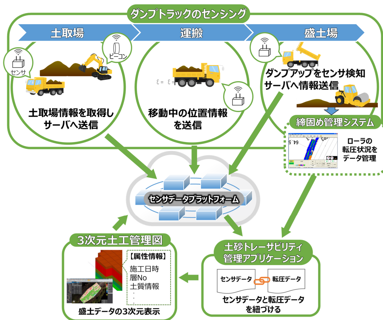
図-1 土砂トレーサビリティ管理システム全体図
