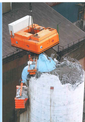
施工状況
