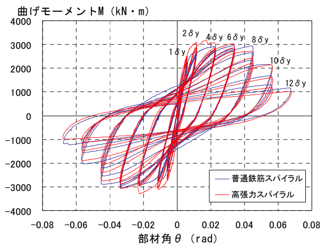
交番載荷試験結果(高張カスパイラル筋との比較)
