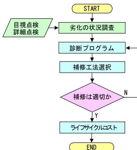
図-2 評価・診断フロー
