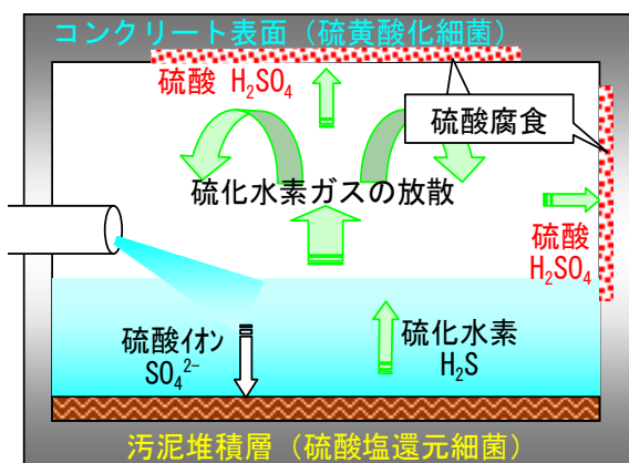
図-1 微生物による硫酸劣化機構
