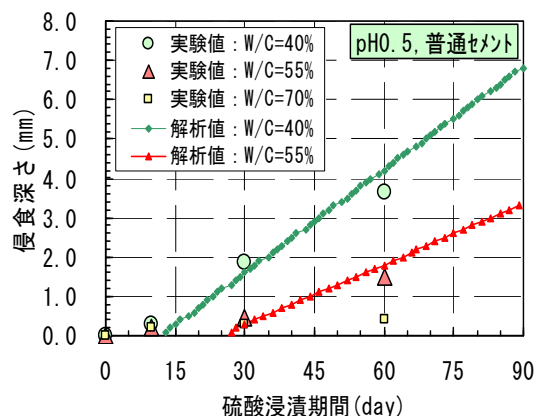
図-5 侵食深さの解析例
