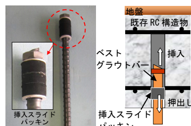
b) 充填入治具と挿入概要
