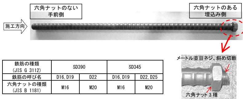
図-2 ベストグラウトバーの概要
