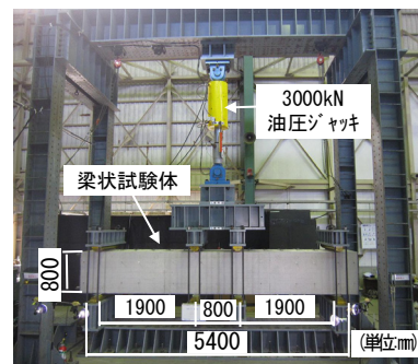
写真-2 梁状試験体の载荷試験
