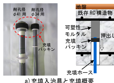
a) 充填入治具と充填概要
