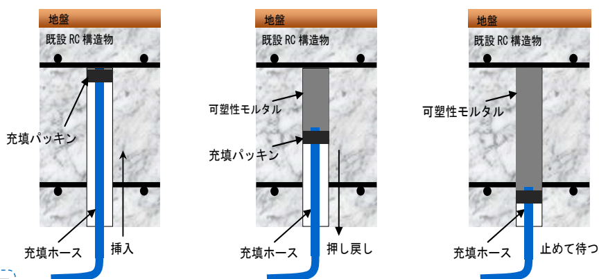
図-6 モルタルの充填手順(上向き施工)
