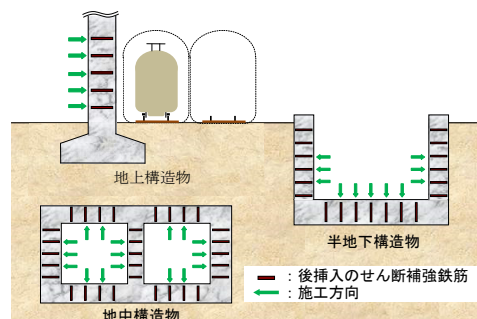
図-3 補強対象構造物の例
