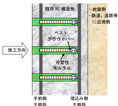
図-1 ベストグラウトバーの施工概要
