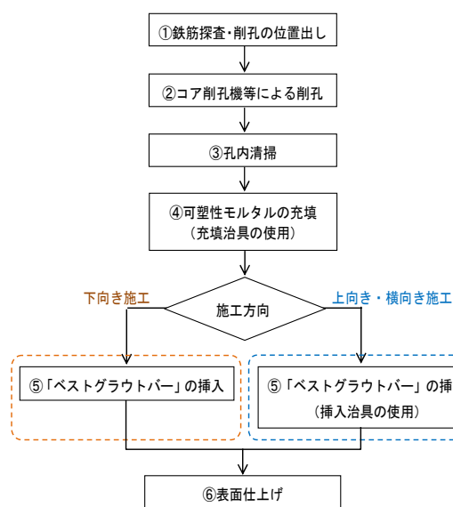
図-5 施工手順
