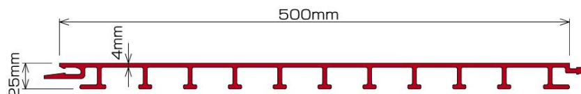
ライニング材の断面形状
