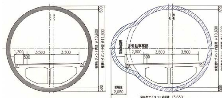
標準部RCセグメント
