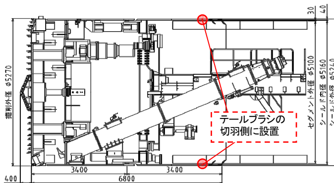
（縦断面図）
