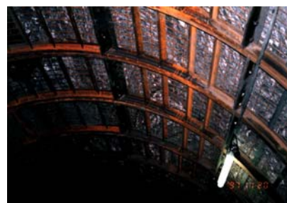
拡張後坑壁に密着したライナー
