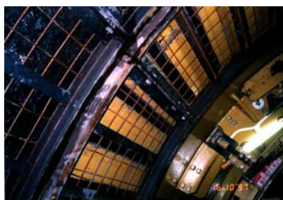
ルーフサポート内でライナー組立
