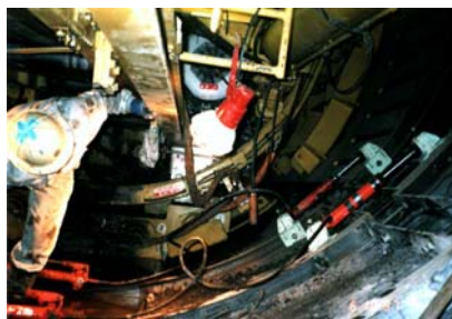
サポート直後でライナー拡張
