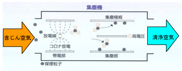
図-1 集じん原理
