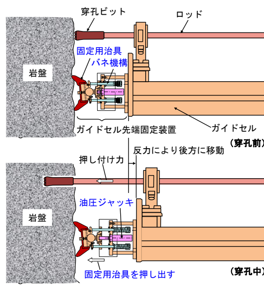
図－２ ガイドセル先端固定装置使用時の穿孔概念図
