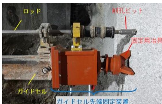
写真－２ ガイドセル先端固定装置の設置状況
