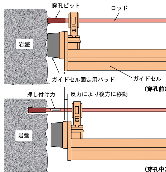
図－１ 通常方法での穿孔概念図
